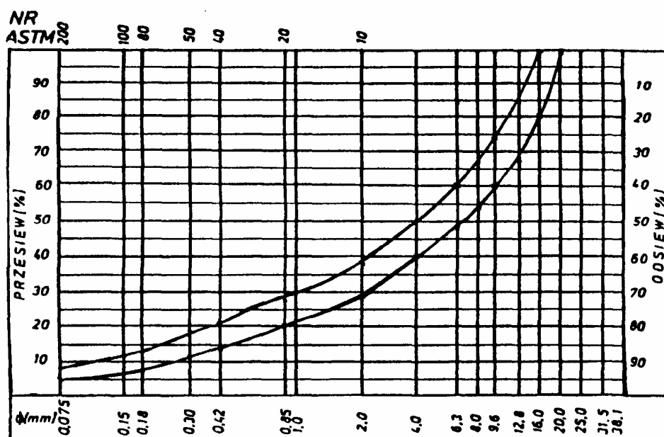
Rys. 1. Krzywe graniczne uziarnienia mieszanki mineralnej 0+20 mm do warstwy ściernicowej z betonu asfaltowego dla KR 3-6
