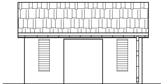
ELEWACJA ZACHODNIA
