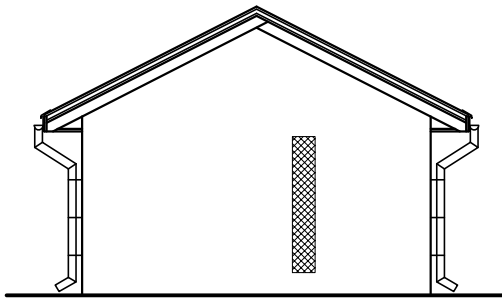
ELEWACJA PÓŁNOCNA
